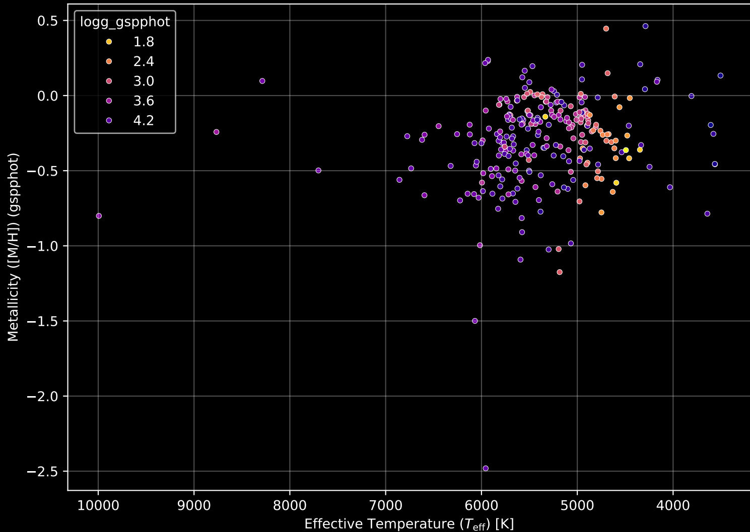
APOGEE DR17 Field: [313+29] Stellar Population Parameters (n= 271)
